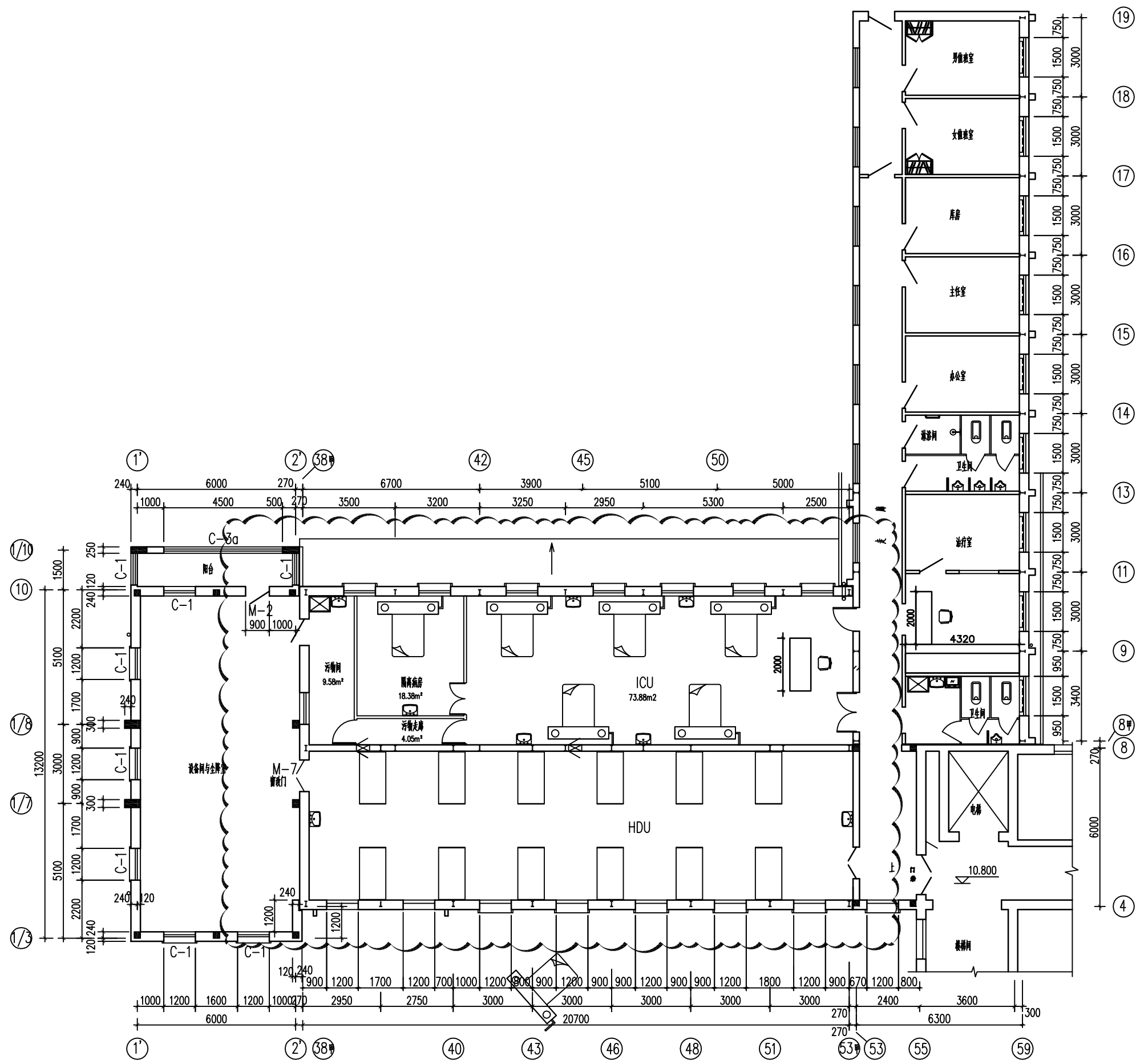
四层平面图 1:100
